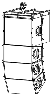
Fig. 6 : Colonne de Q1/Q-SUB en Line Array
